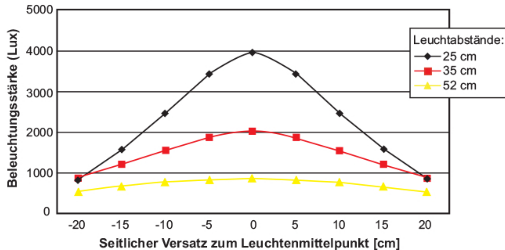
Beleuchtungsstärke in Abhängigkeit vom Abstand
